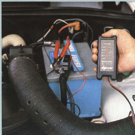
Batterietester
